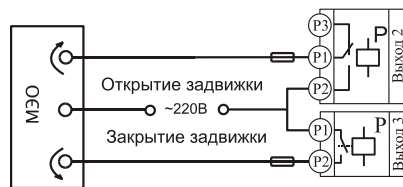
Подключение электродвигателя
